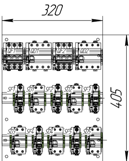
Монтажная плата 2-го уровня
